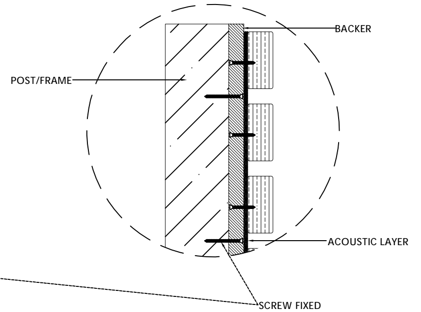
DETAIL 'B-B' SCALE:1:3
